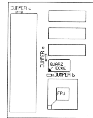
Avantiplatine
