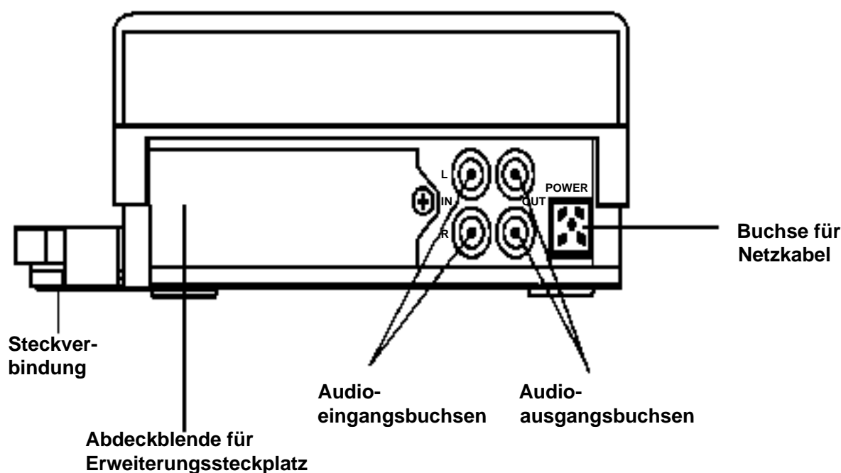
Rückansicht des CD-ROM-Laufwerks
